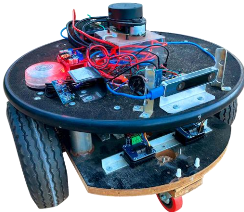
ROBOT AGRÍCOLA MULTIPROPÓSITO Primera aplicación: fumigación de viveros.
